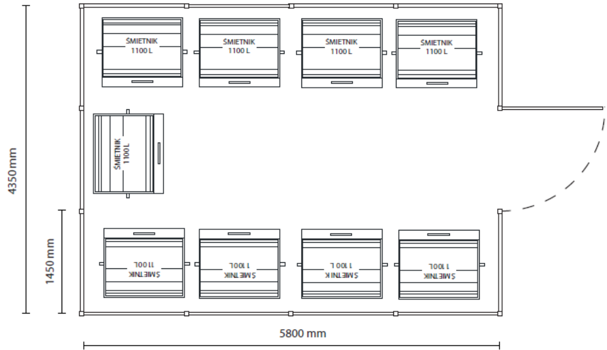
Układ pojemników i wymiary wiaty
